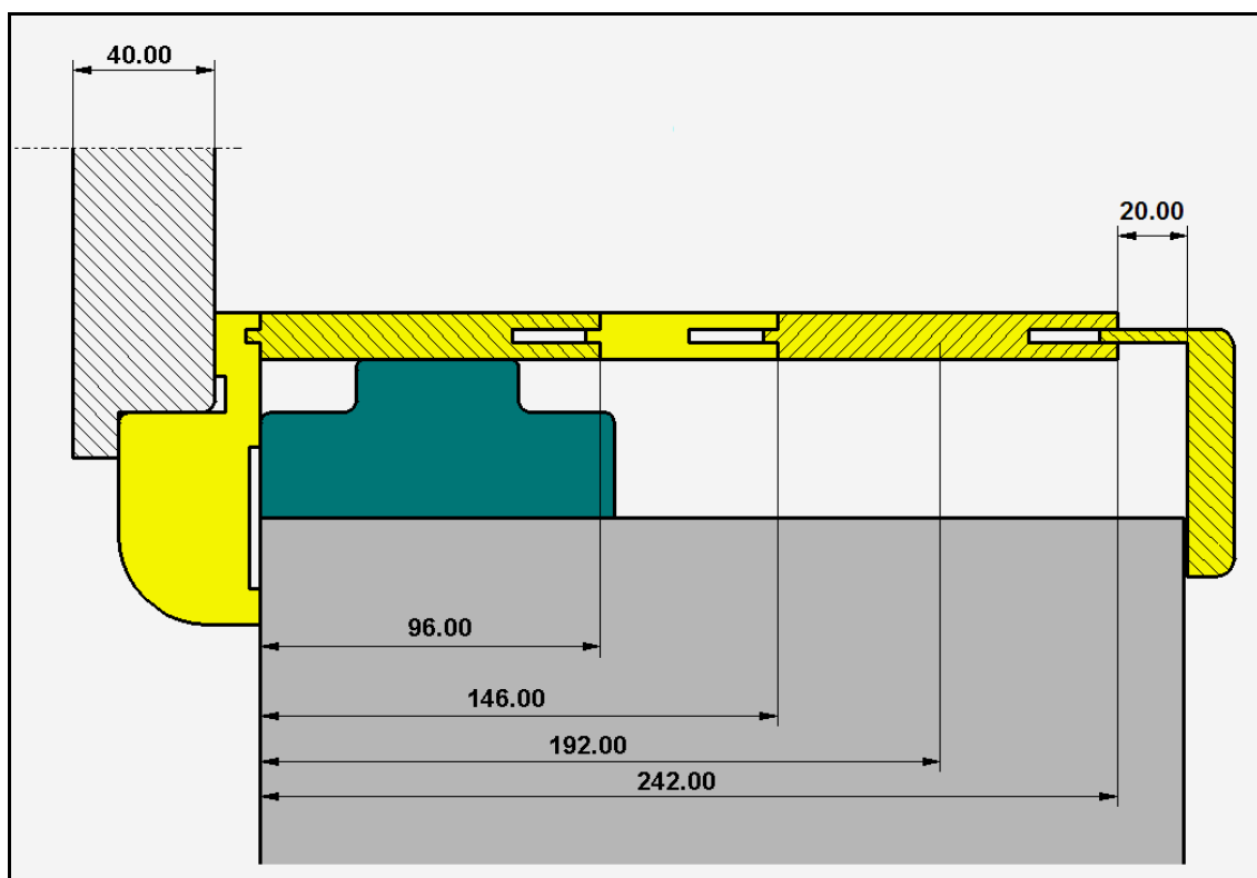
Rysunek 2. Ościeżnica zakrywająca całą grubość muru.
