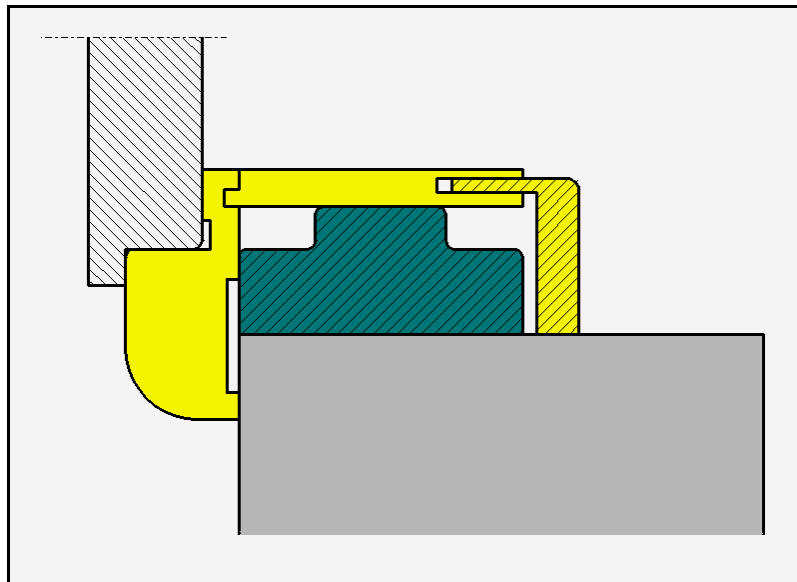
Rysunek 1. Ościeżnica zakrywająca - standardowa.
